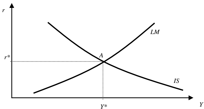
Рис. 1. Равновесие на товарном и денежном рынках в модели IS-LM
